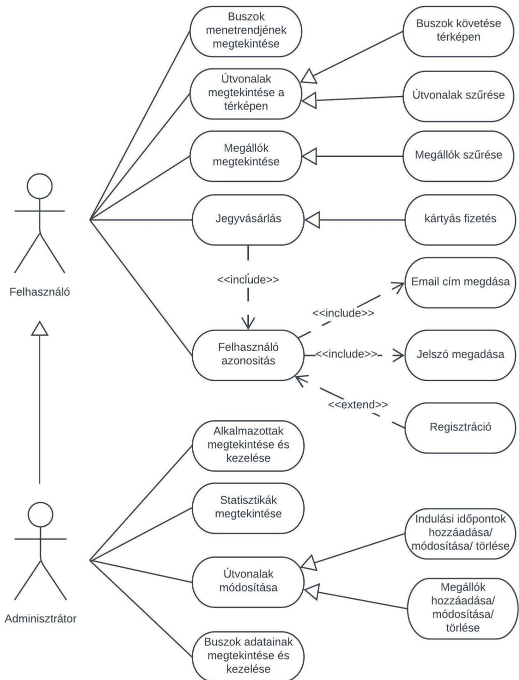
3.1. ábra. Use-case diagram a felhasználók és az adminisztrátorok lehetőségeiről
